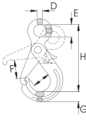
Säkerhetskrok.
