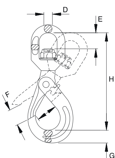
Säkerhetskrok, lekare.
